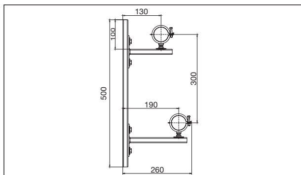
Maße Konsole
