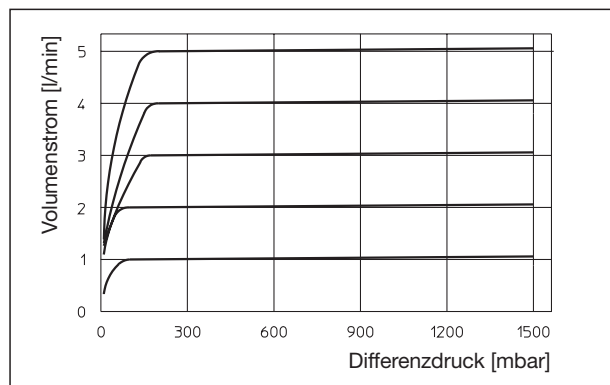
Ventilkennlinien bei verschiedenen Handrad-Voreinstellungen im Vollastbetrieb
