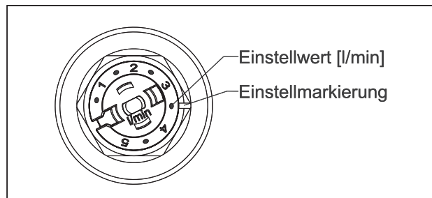
Durchflusseinstellung
