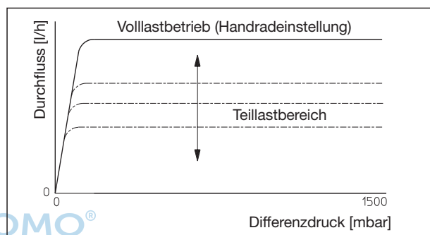
Ventilkennlinien im Teillastbetrieb
