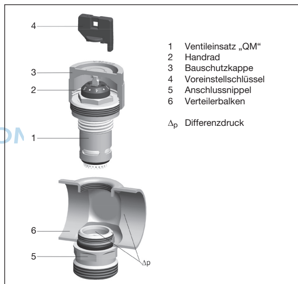
Aufbau Ventileinsatz „QM“
