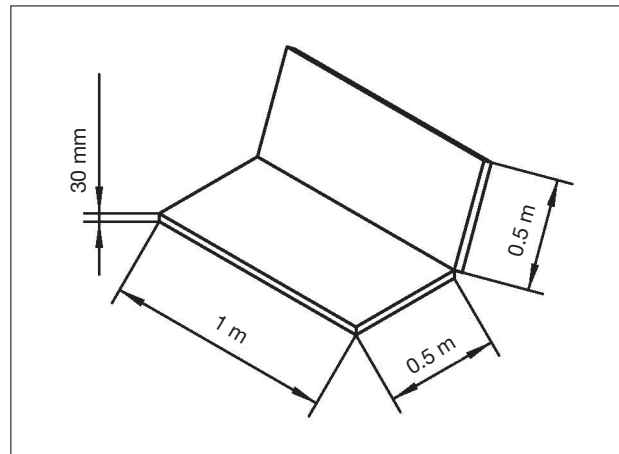
Maße Ausgleichselement 30 mm für Noppenplatte NP-30
