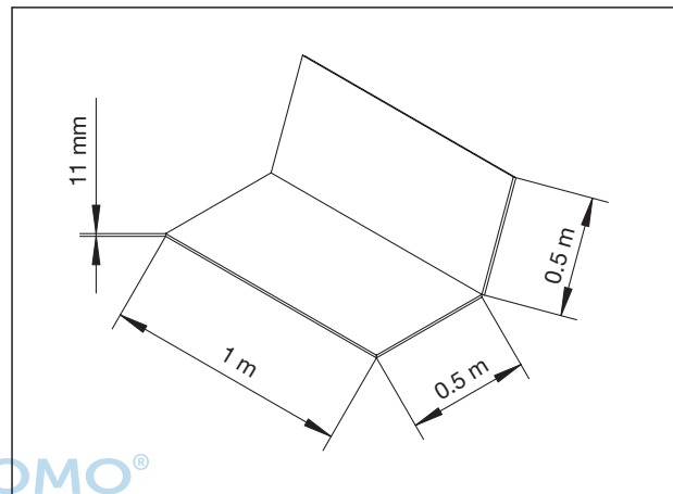
Maße Ausgleichselement 11 mm für Noppenplatte NP-11
