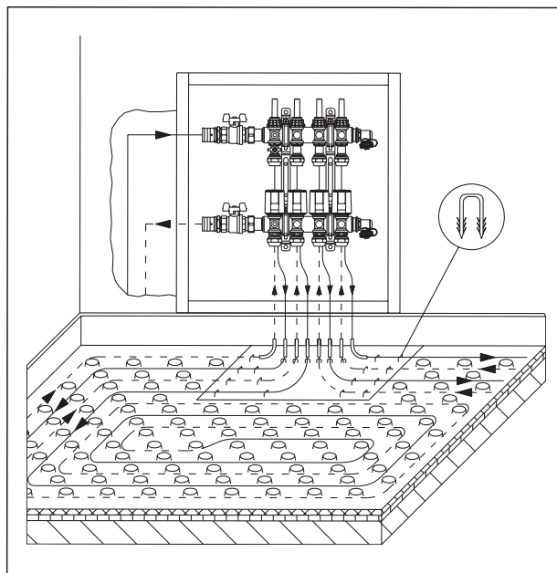
Verlegen der „Copex“, „Copert“ oder „Copipe“ Rohre, System Noppenplatte
