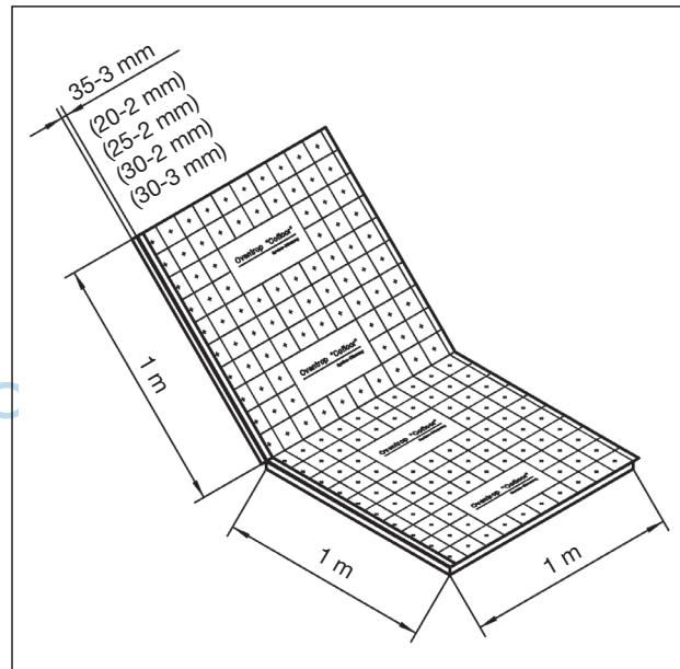
Maße Faltplatte
