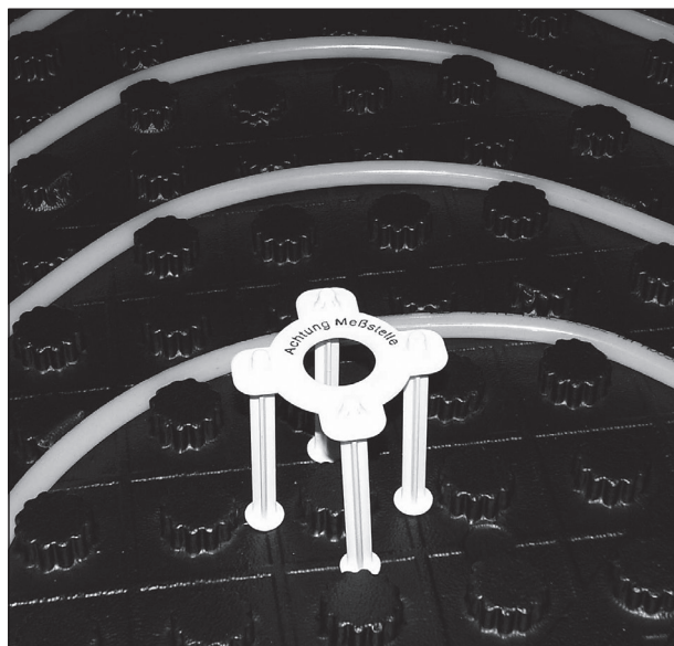
Messstellen-Markierung
