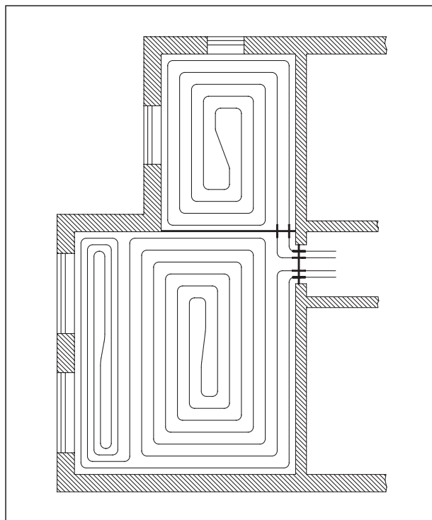
Aufteilung der Heizkreise, Lage von Dehnungsfugen
