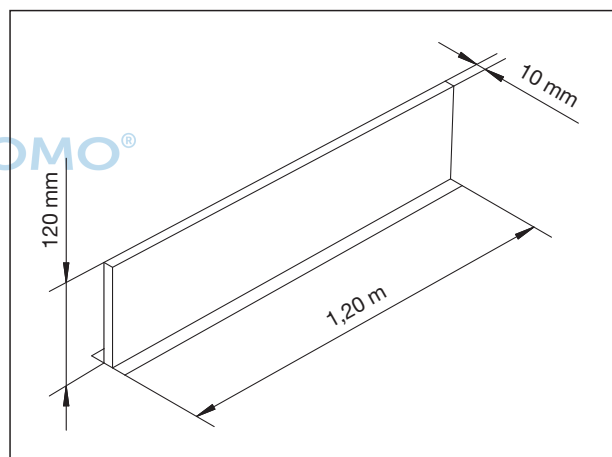
Maße Dehnungsfugenprofil
