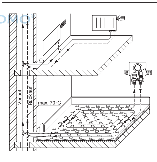
„Cofloor“ Flächenheizungs-System mit „Unibox“ Wandeinbauset
