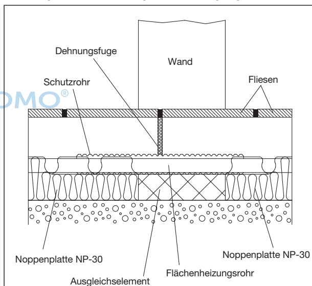
Dehnungsfuge in Türdurchgang
