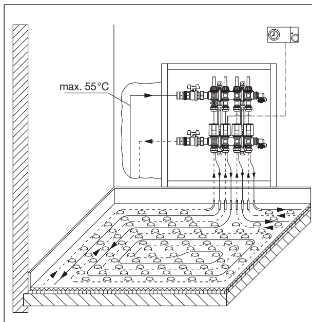
„Cofloor“ Flächenheizungs-System mit „Multidis“ Edelstahl-Verteiler
