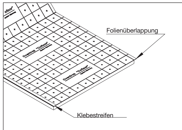
Folienüberlappung und Klebestreifen an Dämmrolle und Faltplatte
