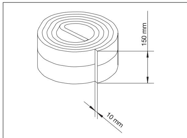
Maße Randdämmstreifen
