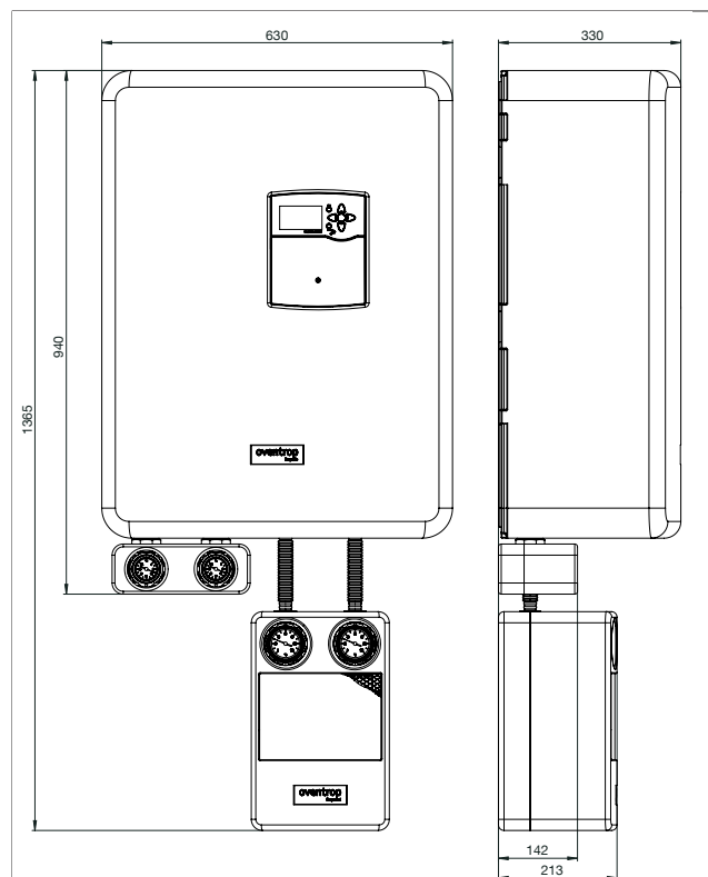
Abb. 3: Abmessungen in mm
