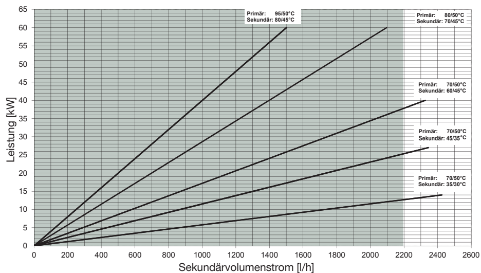
Abb. 8: Leistungsdiagramm; empfohlener max. Volumenstrom Regudis H in Verbindung mit Regumat M 3
