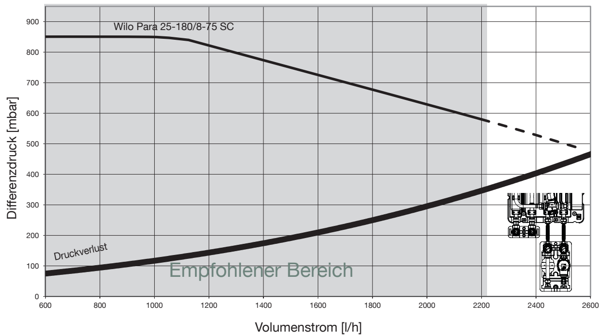
Abb. 5: Druckverlust Sekundärkreis Regudis H-M
