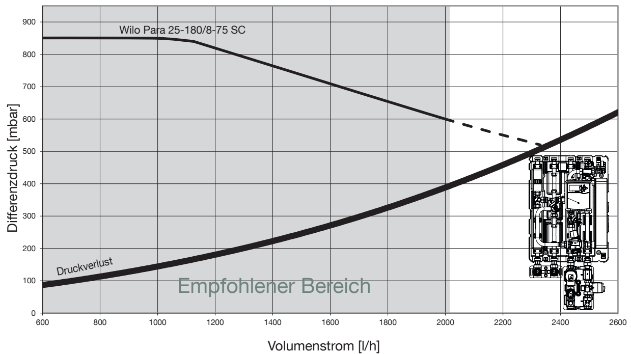
Abb. 5: Druckverlust Sekundärkreis Regudis H-HT
