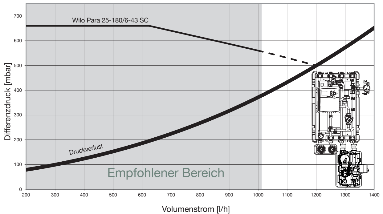
Abb. 5: Druckverlust Sekundärkreis Regudis H-HT
