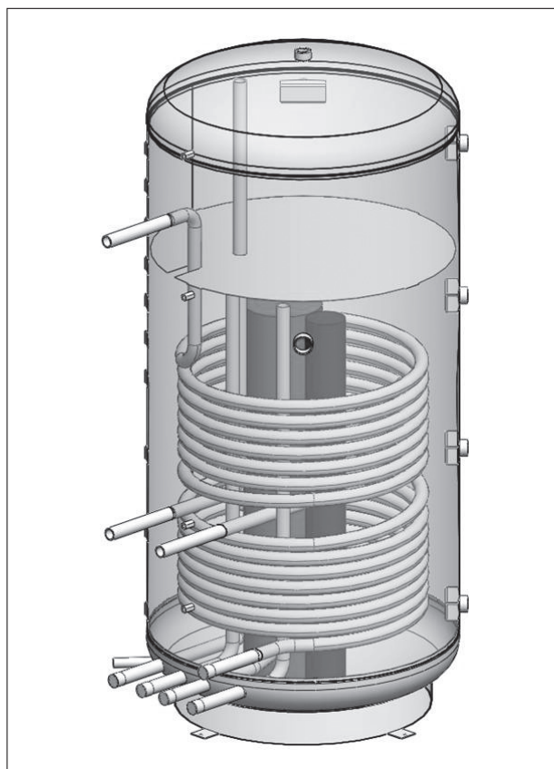
Solarer Pufferspeicher
