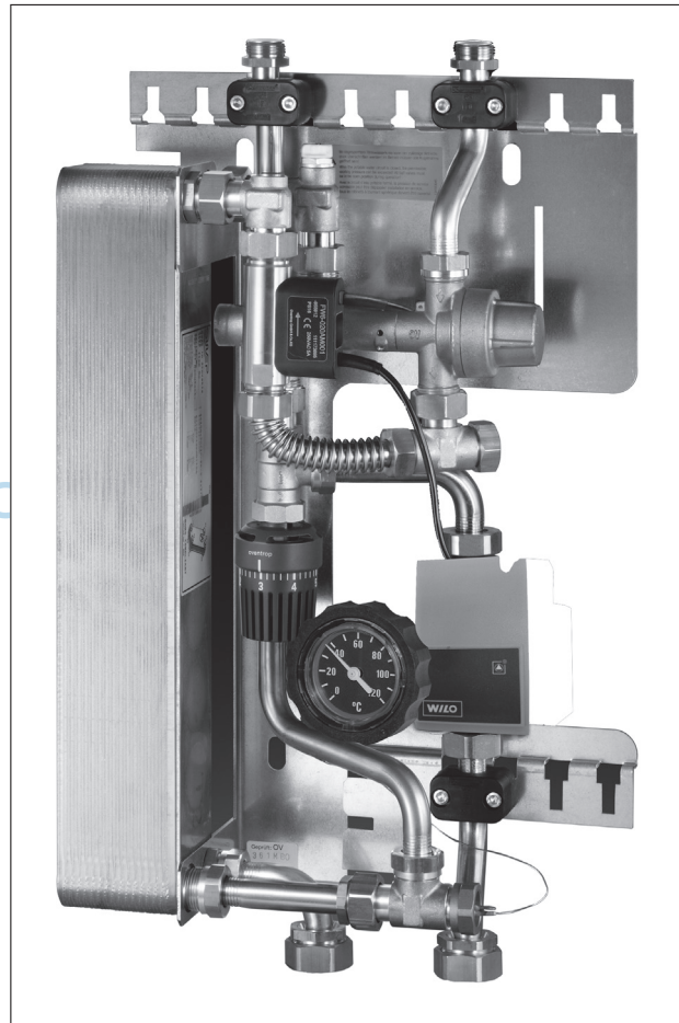
Anbaugruppe Frischwasser
