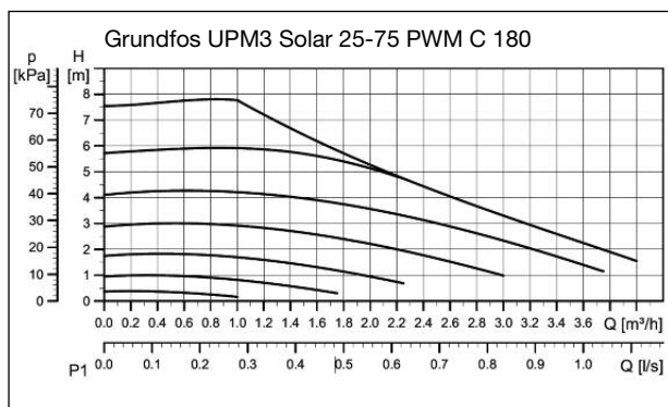
Pumpenkennlinien
