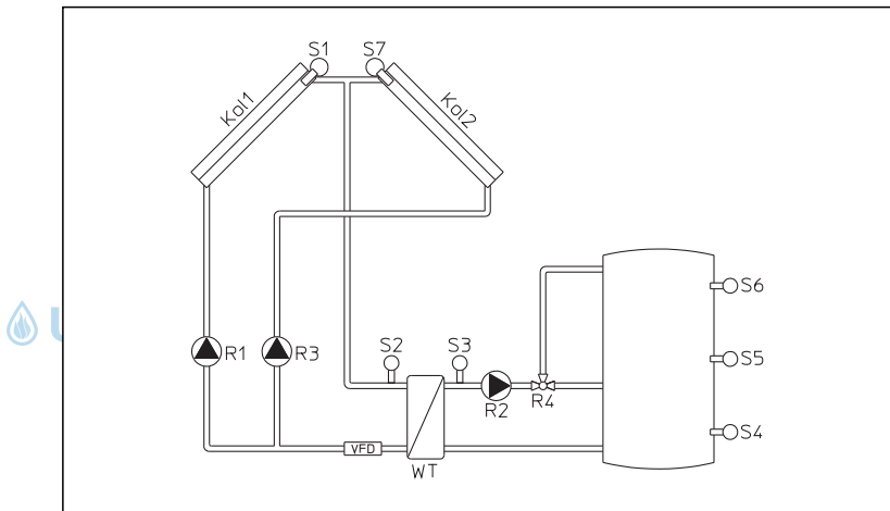
Für 2 Kollektorfelder mit Speicheranschluss im Schichtladebetrieb
