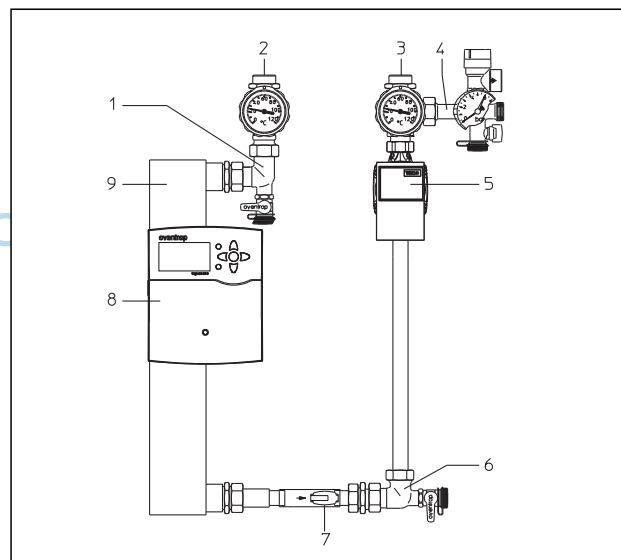
Primärkreis „Regusol X-Uno 25“ (vordere Armaturenebene)
