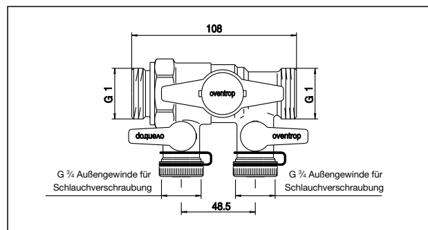
Maße „Regusol“ FSA-Befüll- und Spüleinrichtung
