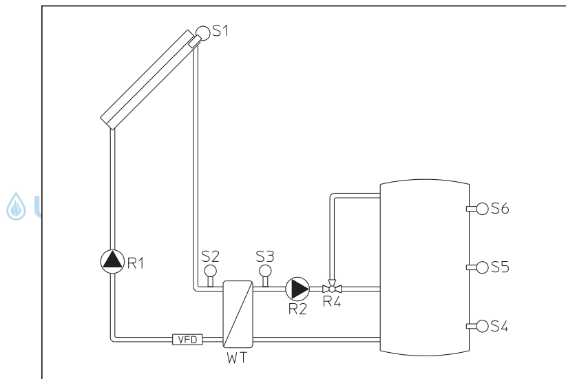
„Regusol X-Duo 25“ – Schichtladung
