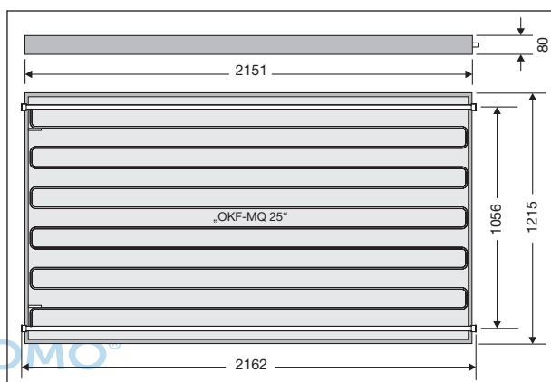
Abmessungen „OKF-MQ25“
