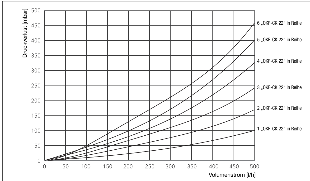
Druckverlustdiagramm OKF-Flachkollektor
