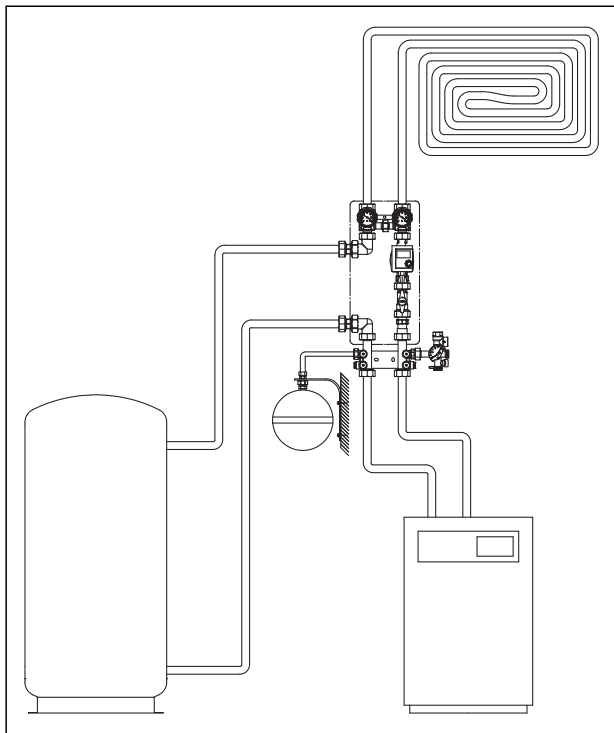
System-Darstellung Pufferspeicher-Anschlussgruppe
