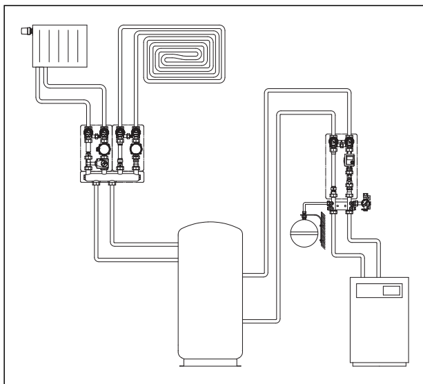
System-Darstellung Heizkreis-Anschlussgruppe
