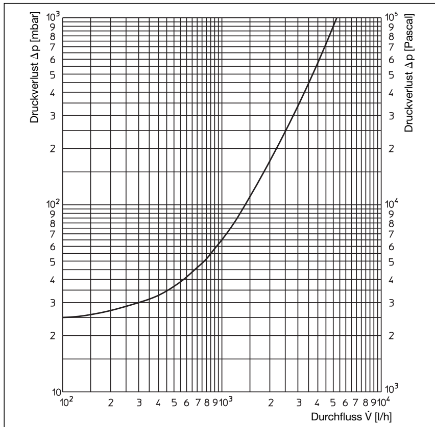
Durchflusssdiagramm „Regumat RTA-180“ DN 32
