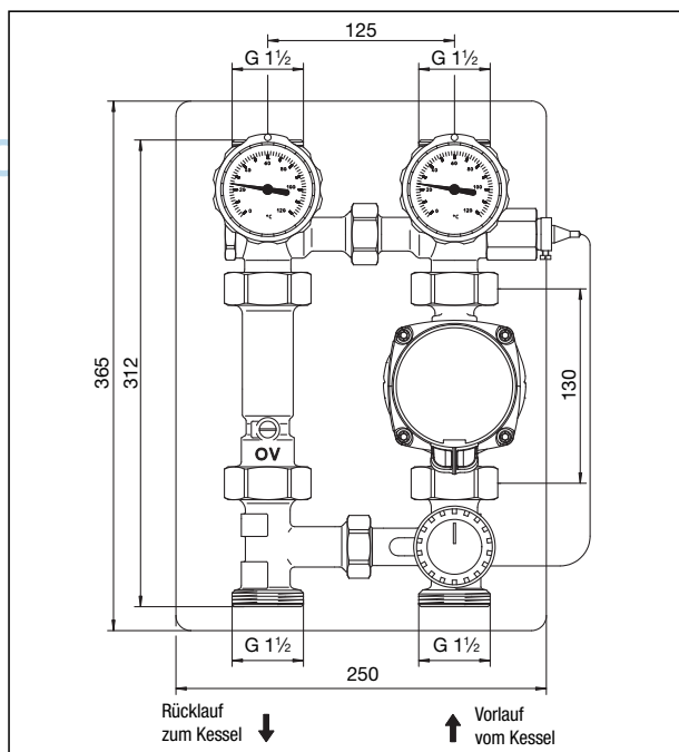
Maße „Regumat F-130“
