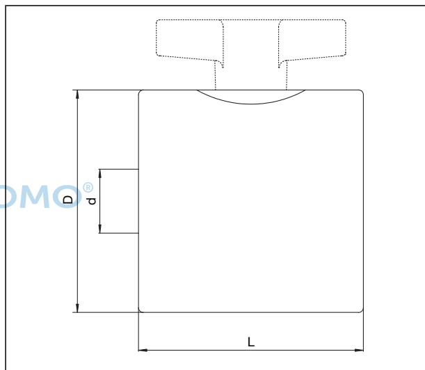
Maße Isolierschalen Artikel-Nr.: 1078x94/95 (DN 25 und DN 32)
