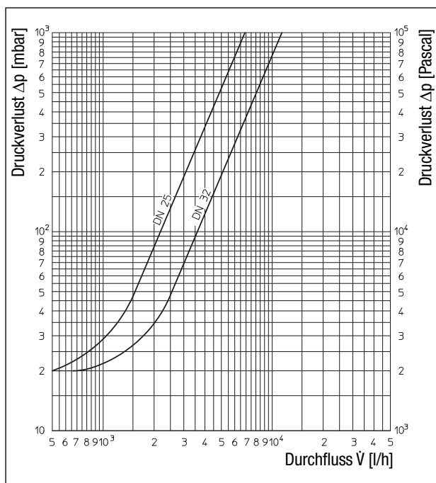
Durchflussdiagramm „Optibal PK“
