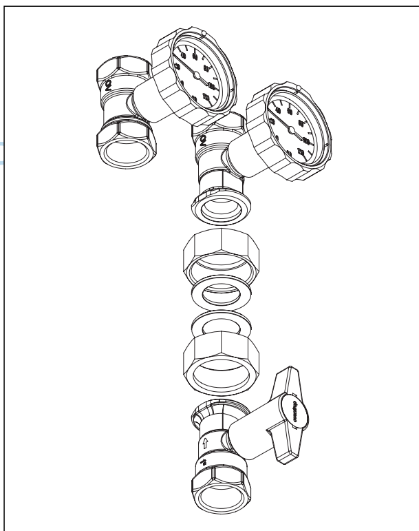
„Optibal PK“ Absperr-Set
