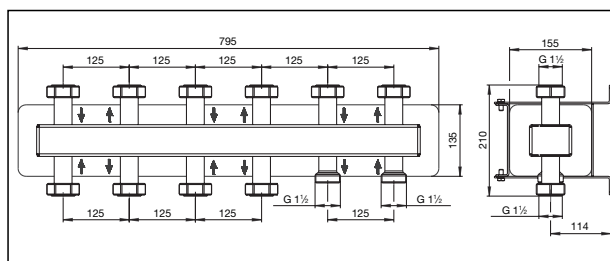
Maße Kompaktverteiler DN 25, 5fach
