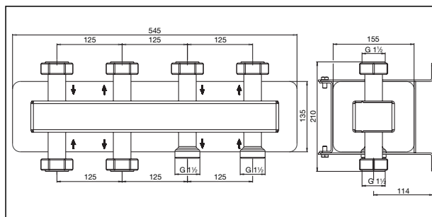
Maße Kompaktverteiler DN 25, 3fach
