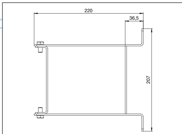
Maße Wandhalterung
