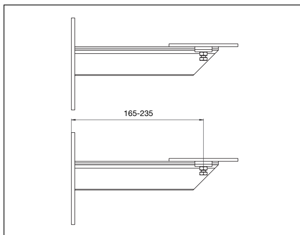
Maße Wandkonsolen-Set
