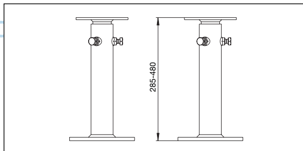
Maße Standkonsolen-Set
