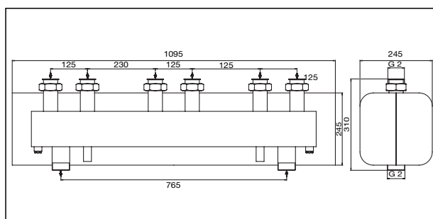
Maße „HydroFixx“ DN 32, 3fach
