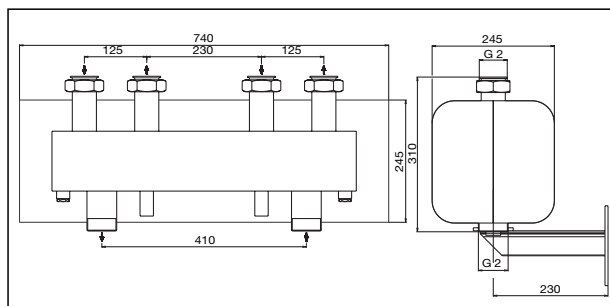
Maße „HydroFixx“ DN 32, 2fach
