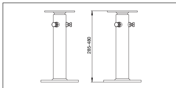
Maße Standkonsolen-Set
