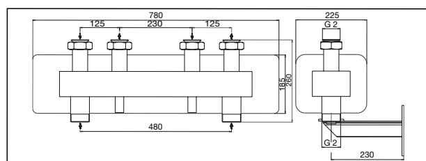
Maße Verteilerbalken DN 32, 2fach
