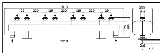
Maße Verteilerbalken DN 32, 4fach
