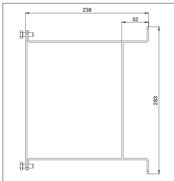
Maße Wandhalterung
