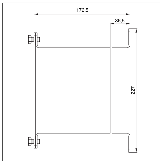
Maße Wandhalterung
