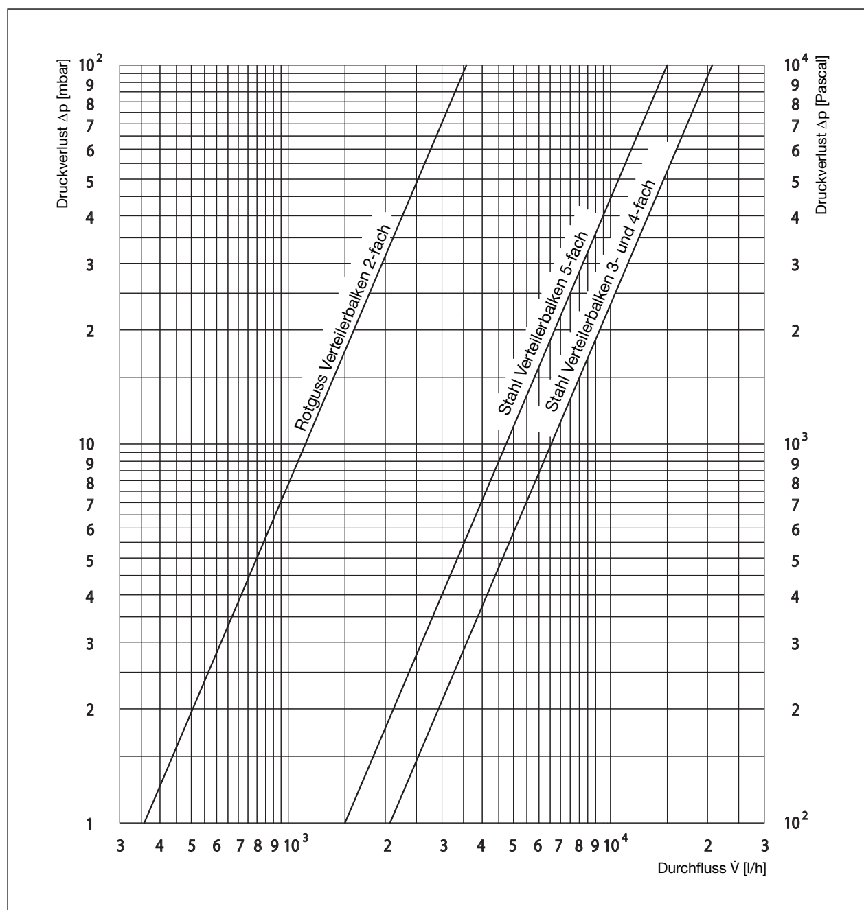
Durchflussdiagramm
