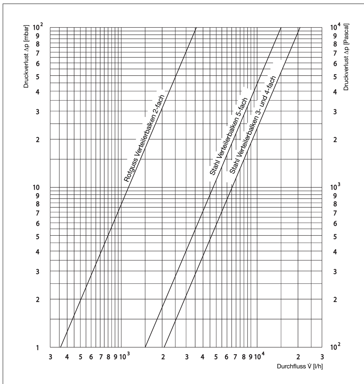
Durchflussdiagramm
