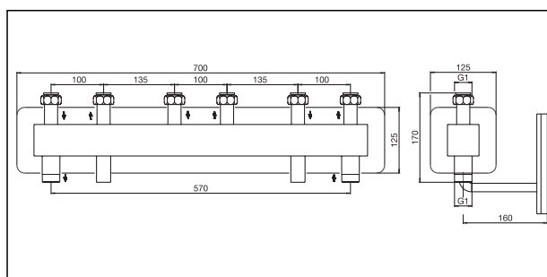
Maße Verteilerbalken DN 20, 3fach
