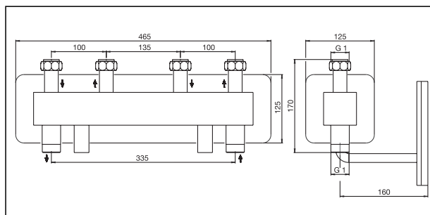
Maße Verteilerbalken DN 20, 2fach
