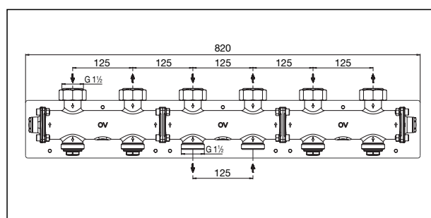
Maße Modulverteiler DN 25, 3fach
