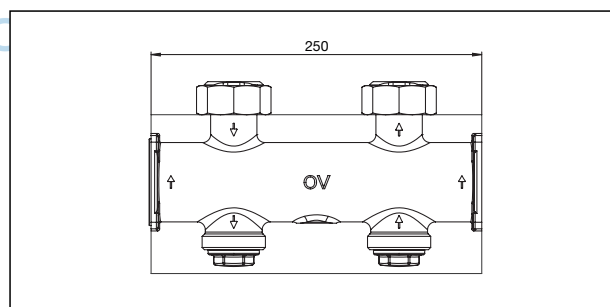
Maße Erweiterungsmodul
