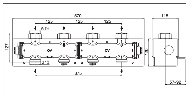
Maße Modulverteiler DN 25, 2fach
