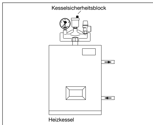
System-Darstellung
