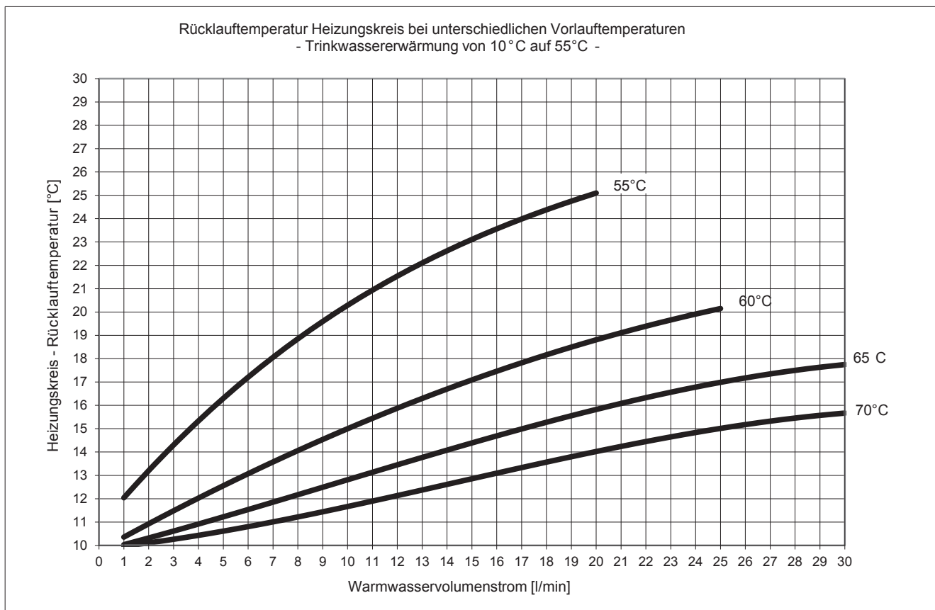
Abb. 31: Leistungsbereich 3, Trinkwassererwärmung auf 55 °C (Leistungsangaben gem. SPF-Prüfprozedur)
