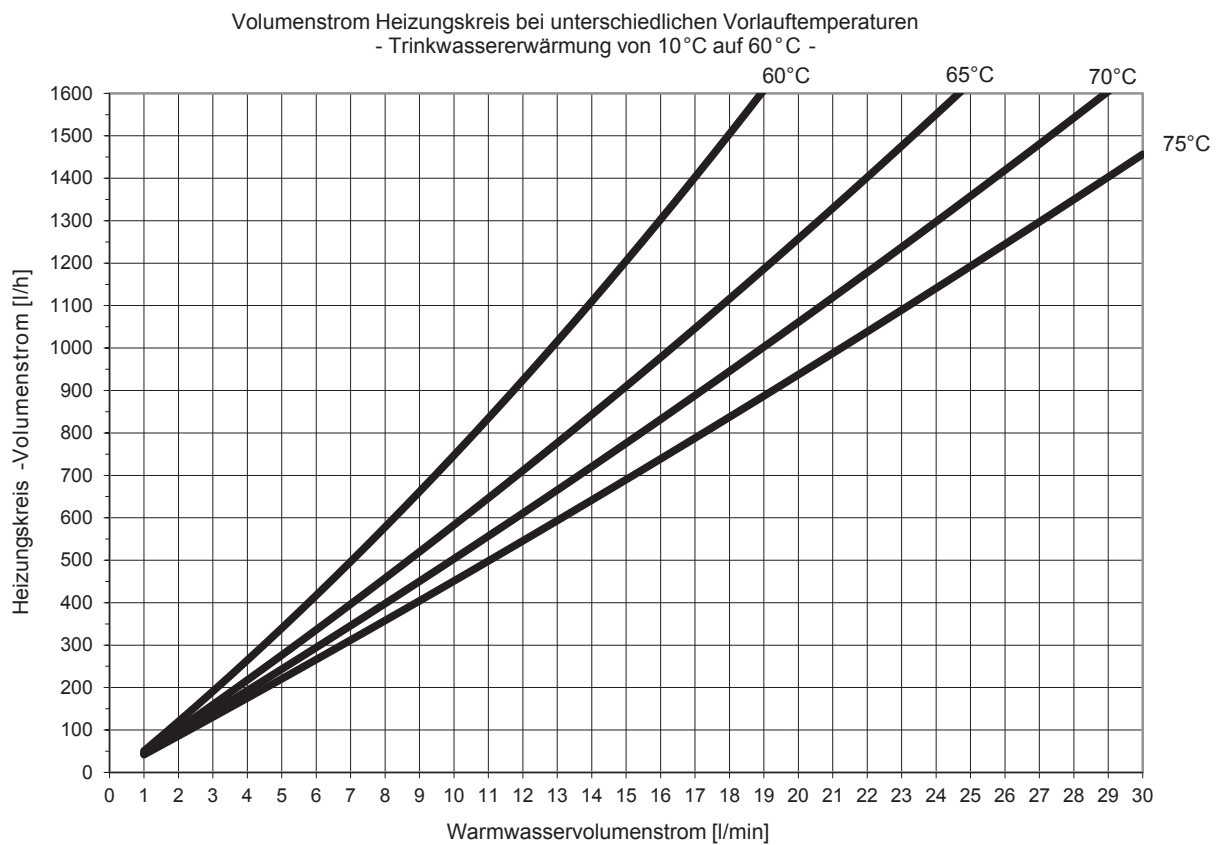
Abb. 32: Leistungsbereich 3, Trinkwassererwärmung auf 60°C (Leistungsangaben gem. SPF-Prüfprozedur)
