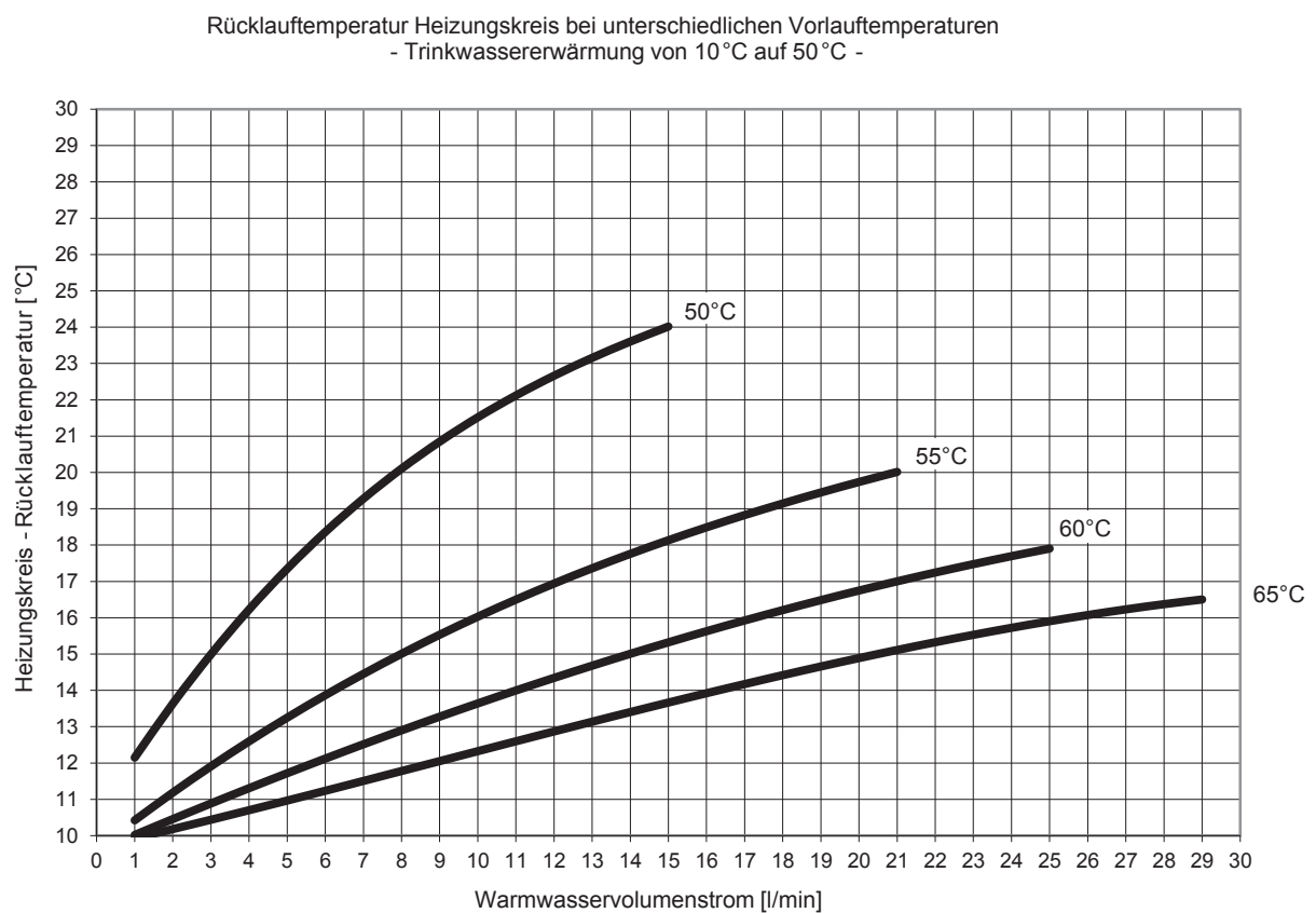
Abb. 21: Leistungsbereich 2, Trinkwassererwärmung auf 50 °C (Leistungsangaben gem. SPF-Prüfprozedur)
