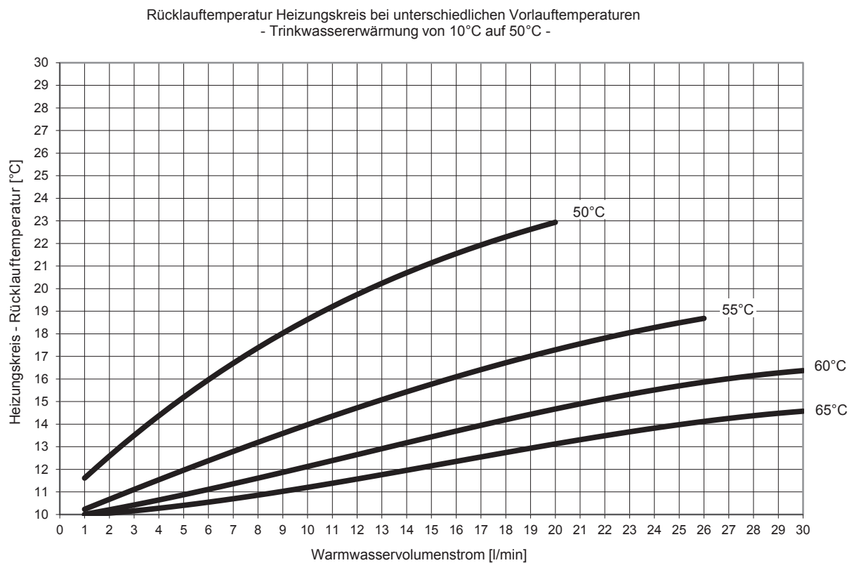
Abb. 29: Leistungsbereich 3, Trinkwassererwärmung auf 50 °C (Leistungsangaben gem. SPF-Prüfprozedur)
