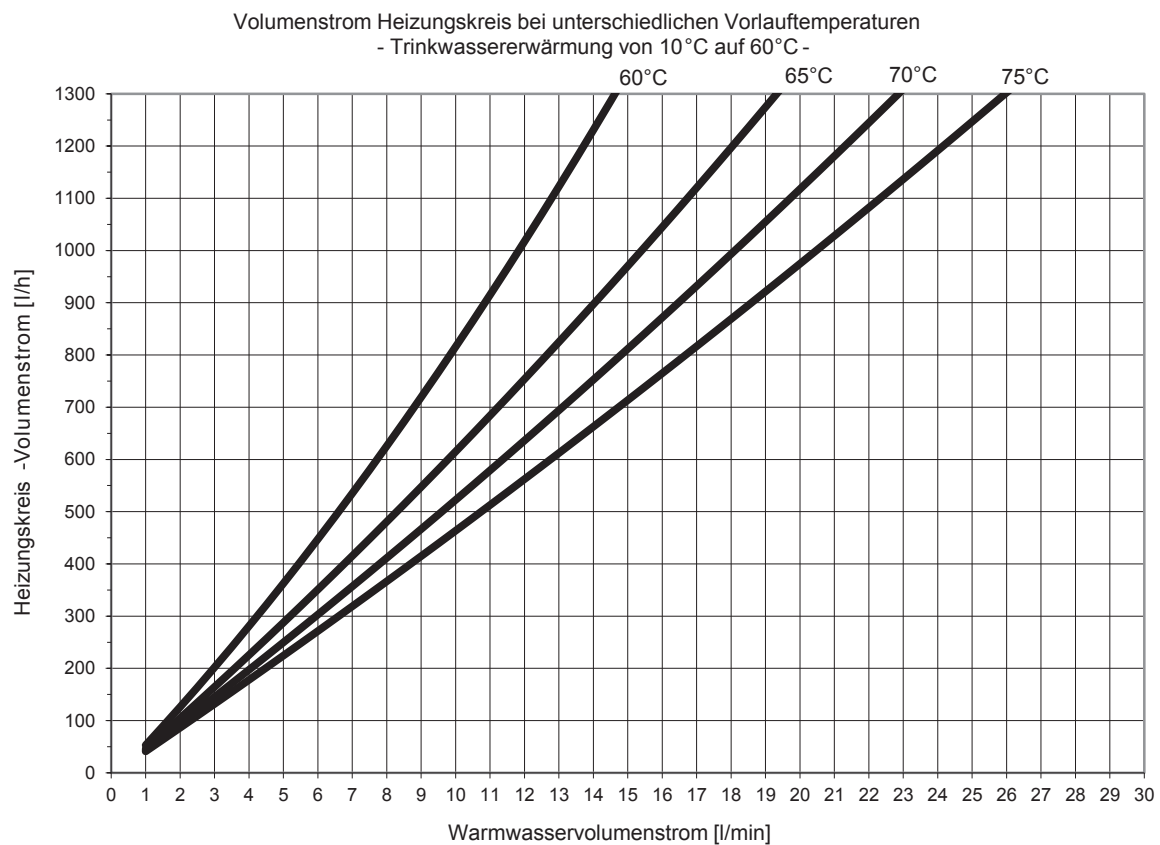
Abb. 24: Leistungsbereich 2, Trinkwassererwärmung auf 60 °C (Leistungsangaben gem. SPF-Prüfprozedur)
