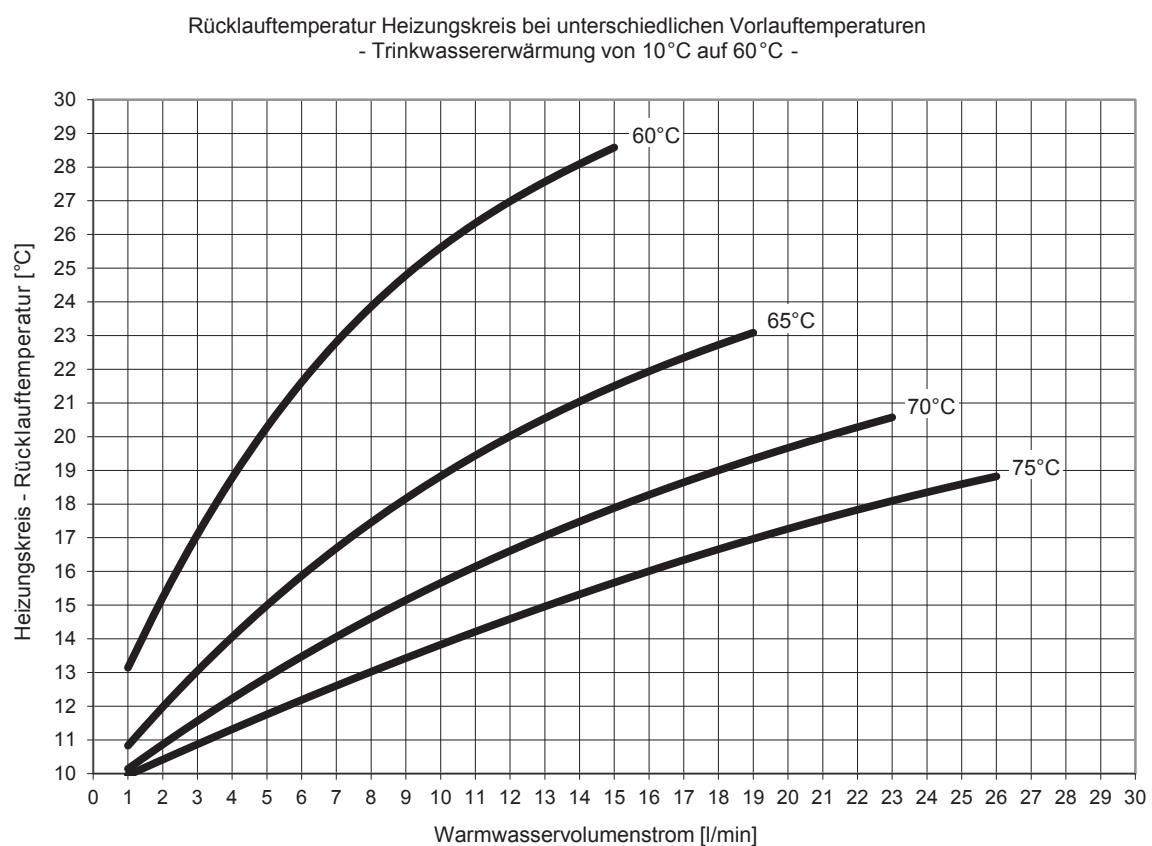
Abb. 25: Leistungsbereich 2, Trinkwassererwärmung auf 60 °C (Leistungsangaben gem. SPF-Prüfprozedur)
