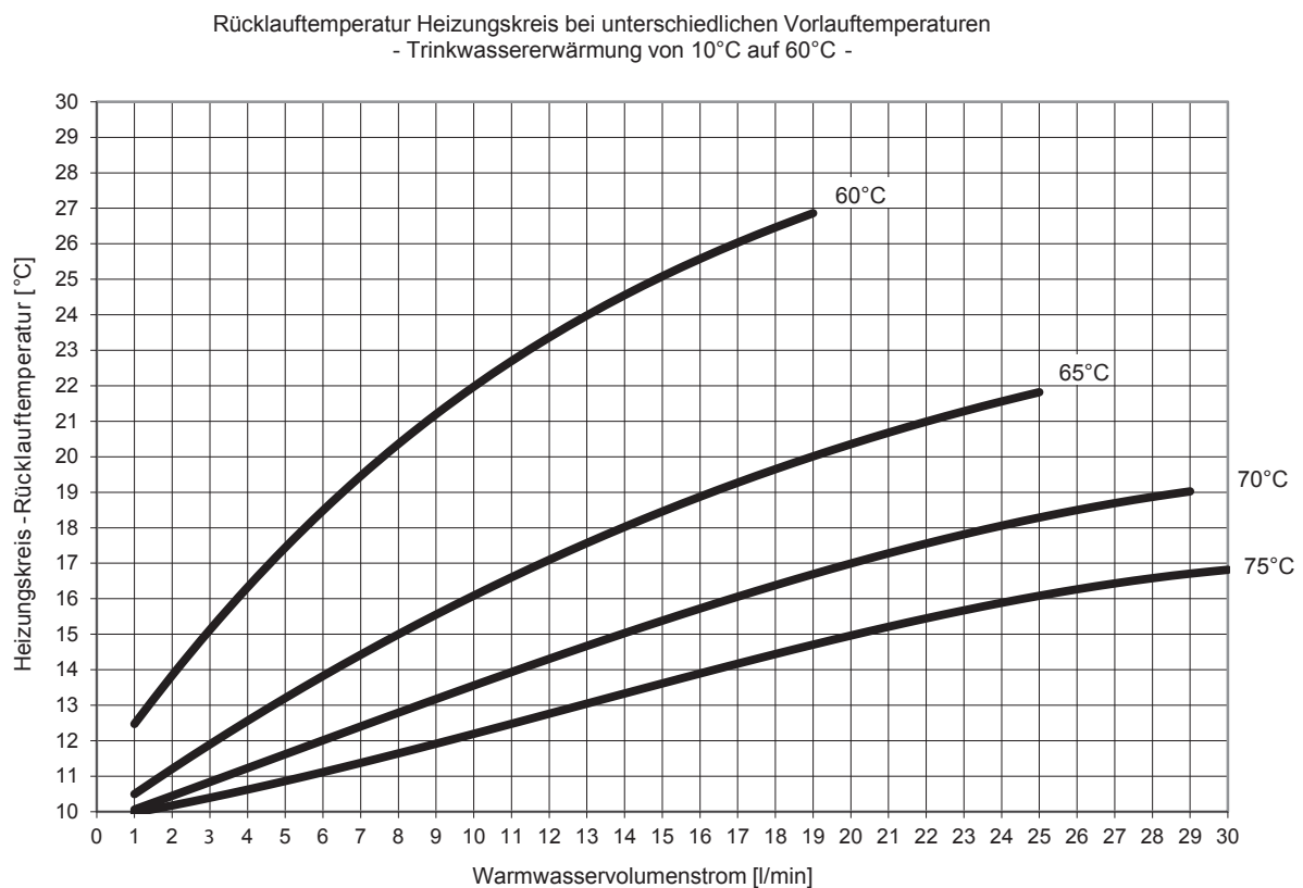
Abb. 33: Leistungsbereich 3, Trinkwassererwärmung auf 60°C (Leistungsangaben gem. SPF-Prüfprozedur)
