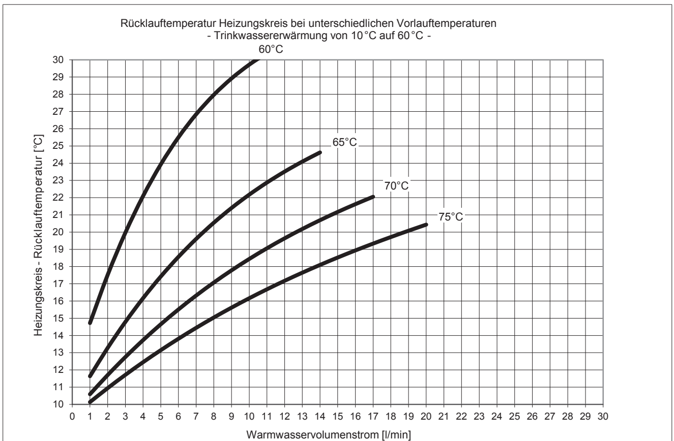
Abb. 17: Leistungsbereich 1, Trinkwassererwärmung auf 60 °C (Leistungsangaben gem. SPF-Prüfprozedur)
