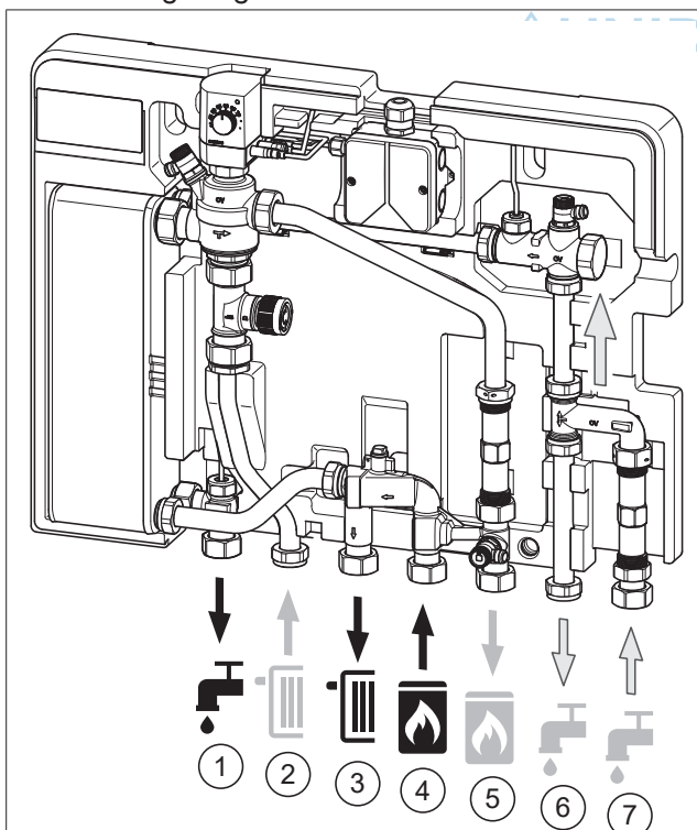
Abb. 1: Anschlussbelegung
