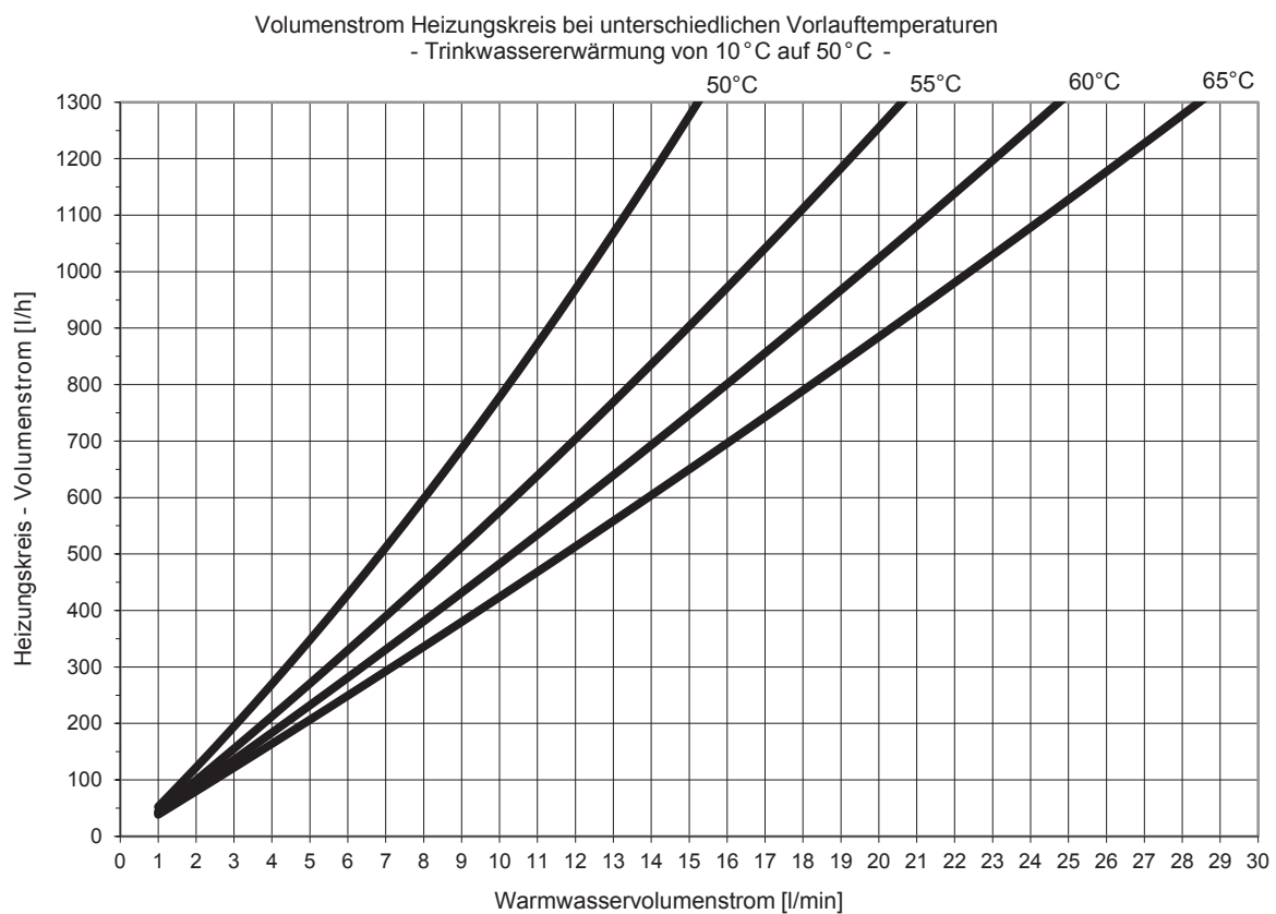
Abb. 20: Leistungsbereich 2, Trinkwassererwärmung auf 50 °C (Leistungsangaben gem. SPF-Prüfprozedur)
