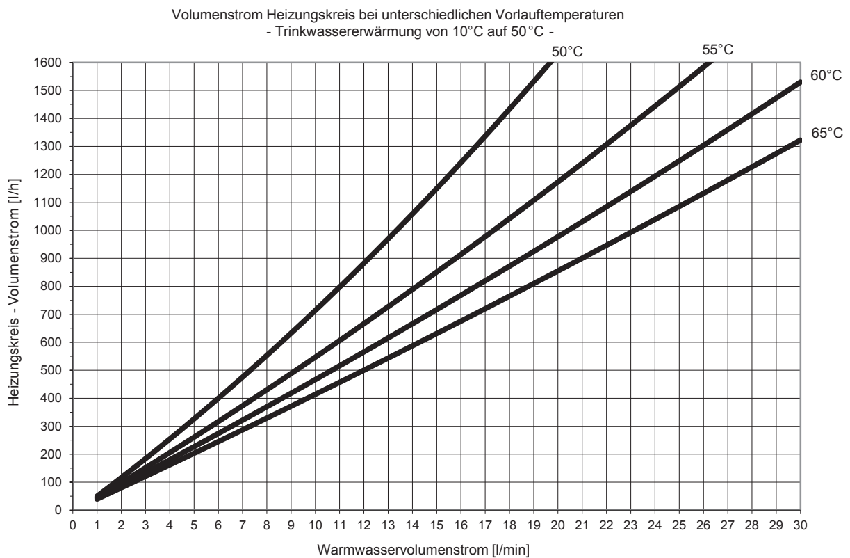
Abb. 28: Leistungsbereich 3, Trinkwassererwärmung auf 50 °C (Leistungsangaben gem. SPF-Prüfprozedur)
