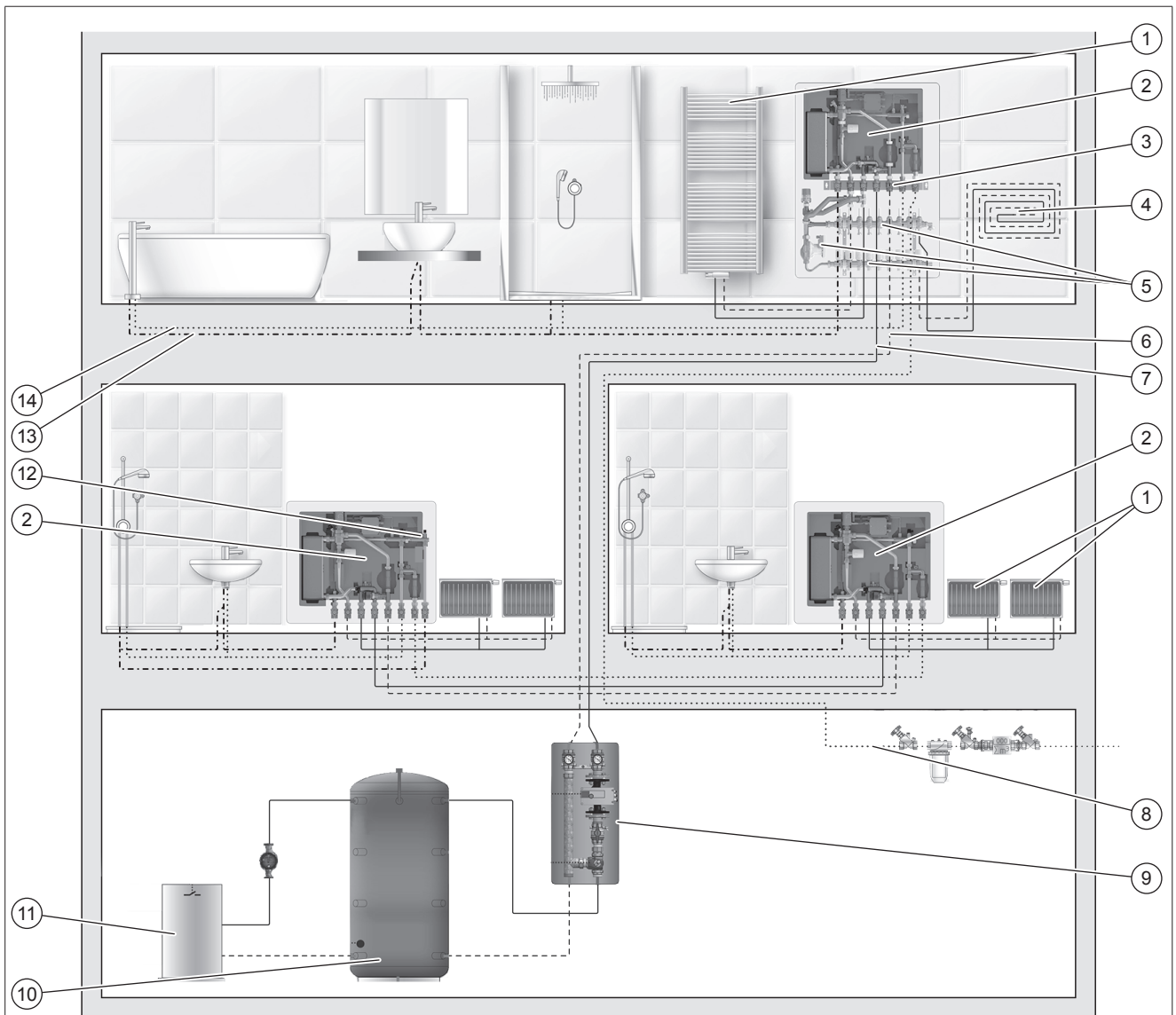
Abb. 5: Anlagenschema: Wohnungsstation
