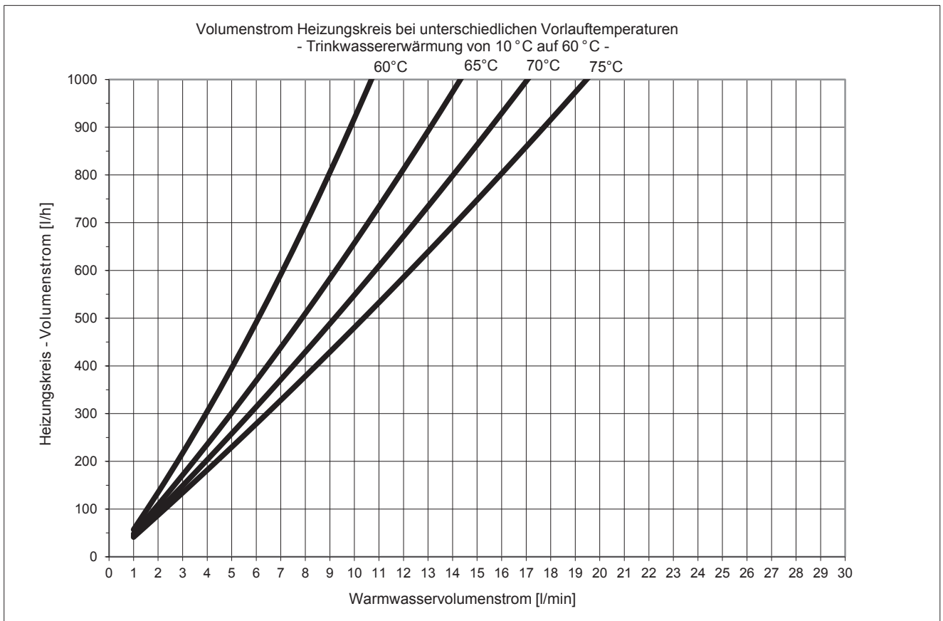
Abb. 16: Leistungsbereich 1, Trinkwassererwärmung auf 60 °C (Leistungsangaben gem. SPF-Prüfprozedur)
