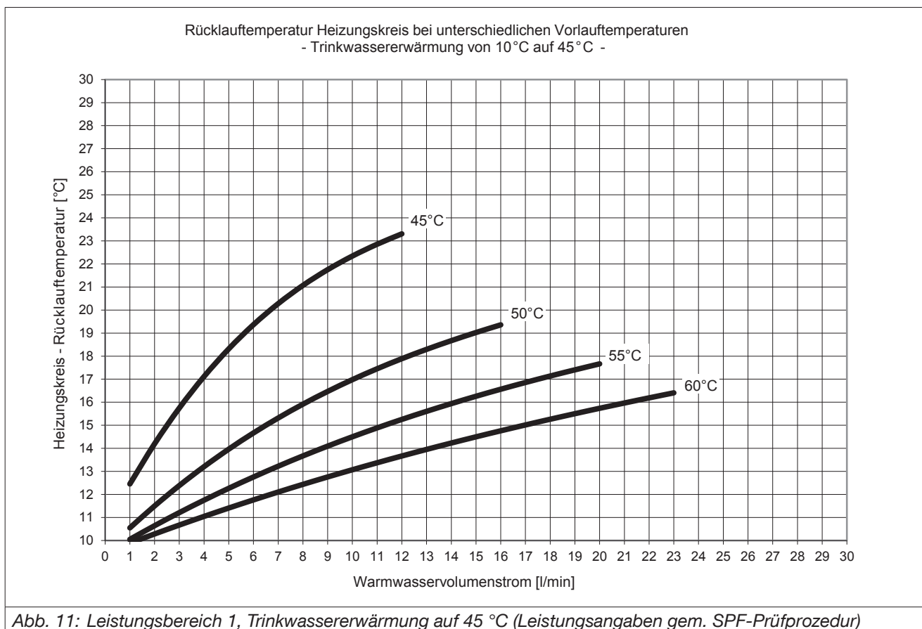
Abb. 10: Leistungsbereich 1, Trinkwassererwärmung auf 45 °C (Leistungsangaben gem. SPF-Prüfprozedur)
