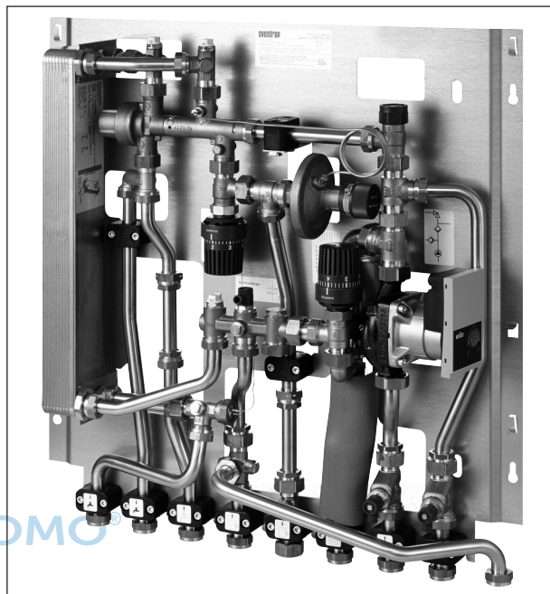
„Regudis W-HTF“ gemischter Heizkreis mit Hochtemperaturkreis
