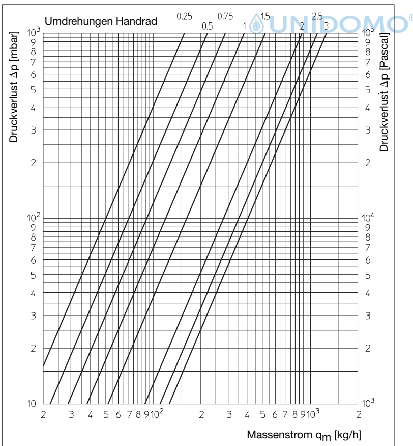
Diagramm: DN 10 - DN 20 Durchgangsventil
