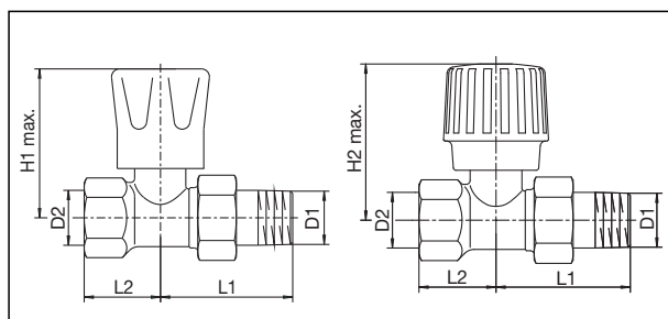
Maße Eckventil
