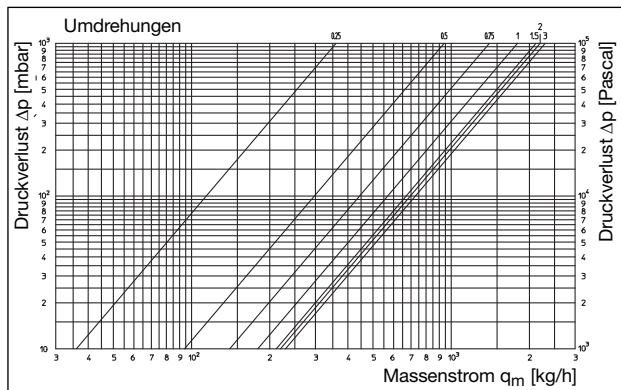
DN 20 Durchgang
