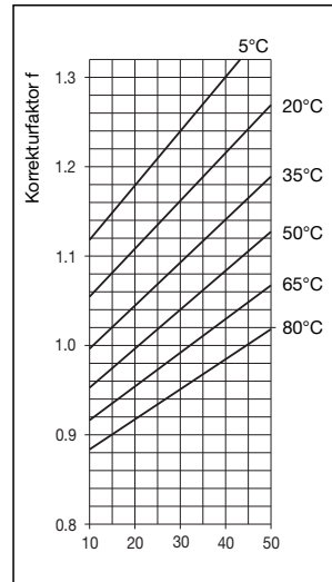
Gewichtsanteil Aethylenglykol [%]
