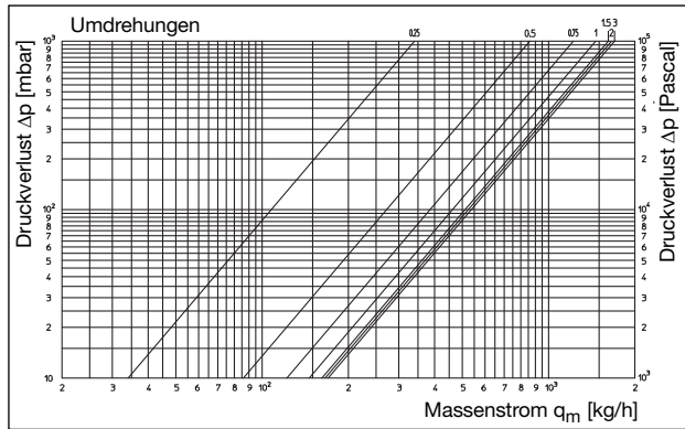
DN 15 Durchgang
