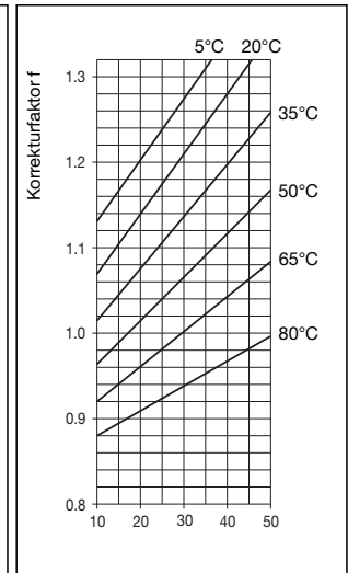
Gewichtsanteil Propylenglykol [%]
