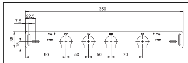
Abmessungen Montagehilfe
