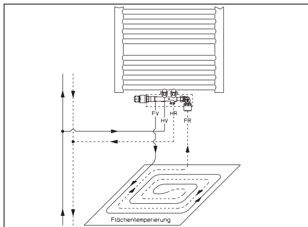
Anschluss-Schema
