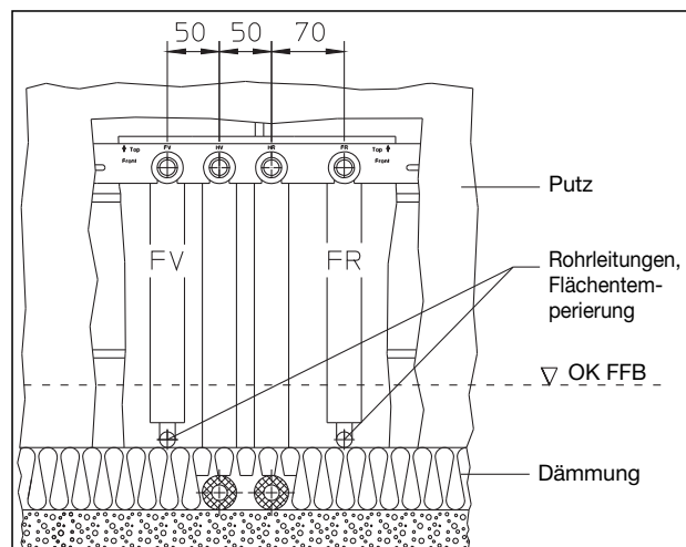
Wandansicht, Flächentemperierung
