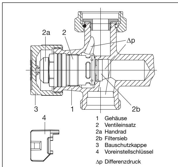
Aufbau Thermostatventil
