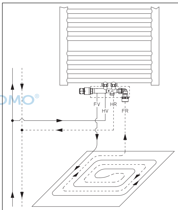
System-Darstellung
