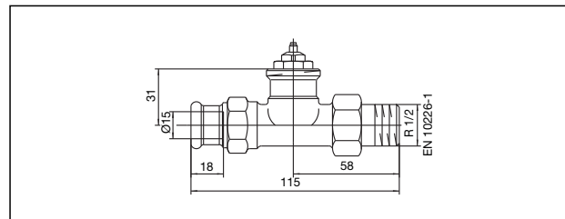
Maße Durchgangsventil
