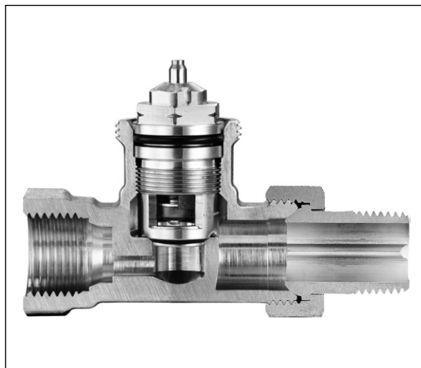
Durchgangsventil „AV 9“
