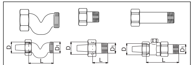
Isolier-Ausgleichs- und Absperrset
