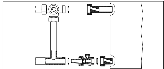
Isolier-Ausgleichs- und Absperrset
