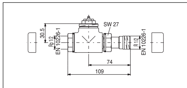
Durchgangsventil
