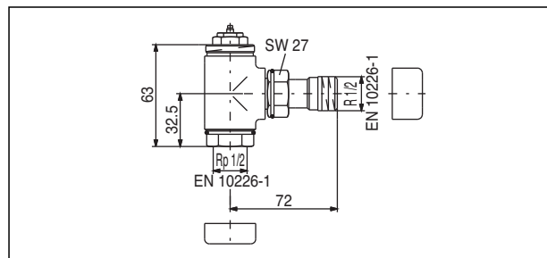
Eckventil
