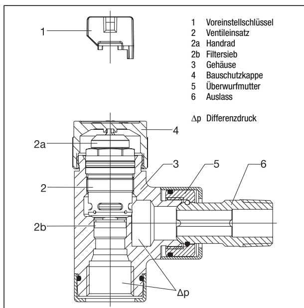
Aufbau Thermostatventil „EQ“
