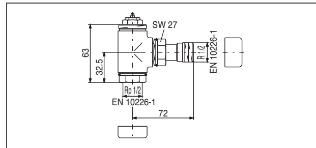
Eckventil
