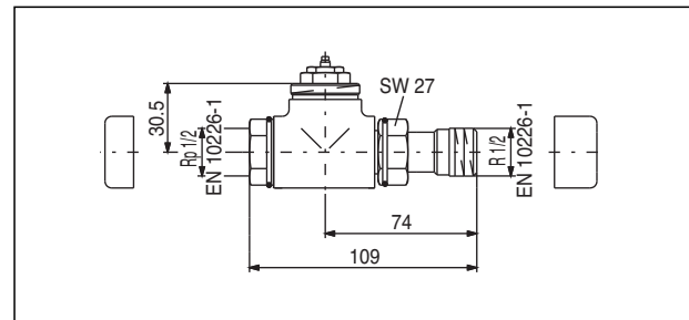
Durchgangsventil
