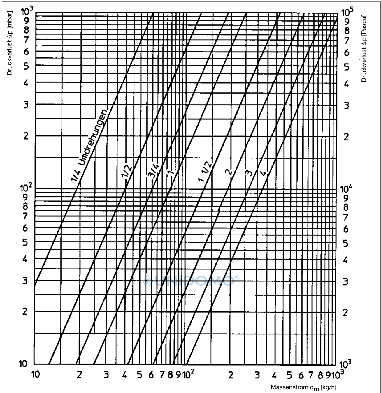
Leistungdaten: Verschraubungen „Combi E“
