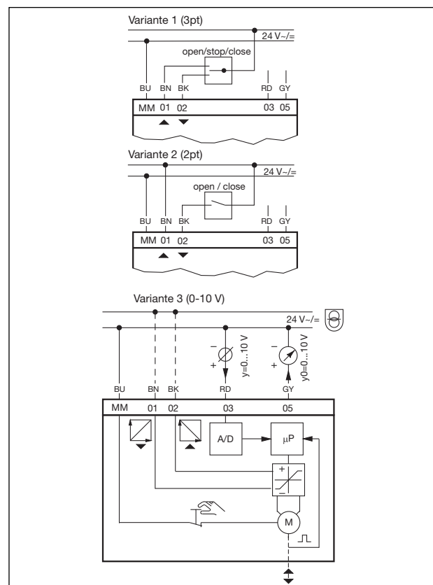
Schaltpläne Artikel-Nr.: 1158010/11
