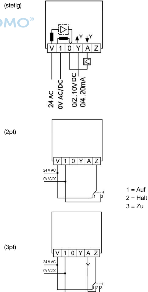
Schaltpläne Artikel-Nr.: 1158021/22
