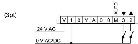
Schaltpläne Artikel-Nr.: 1158020
