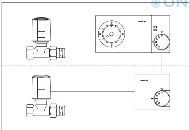
Anschlussbeispiel 3
