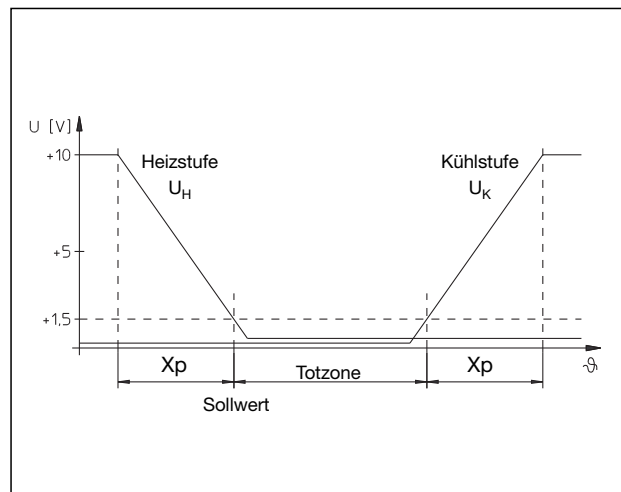
Funktionsdiagramm
