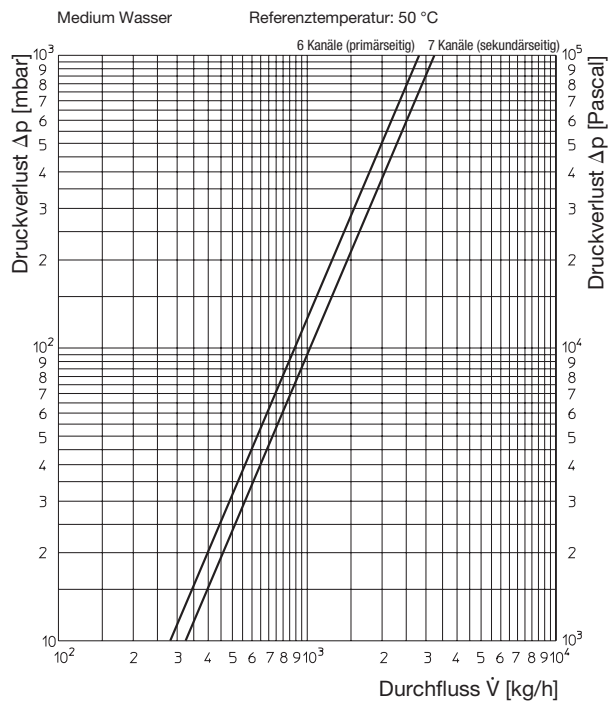
Diagramm Wärmeübertrager
